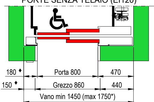
PIANTA VANO CORSA PORTE SENZA TELAIO (EI120)
