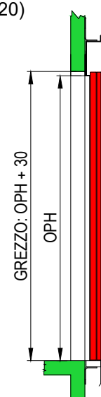
SEZIONE PORTE SENZA TELAIO (EI120)
